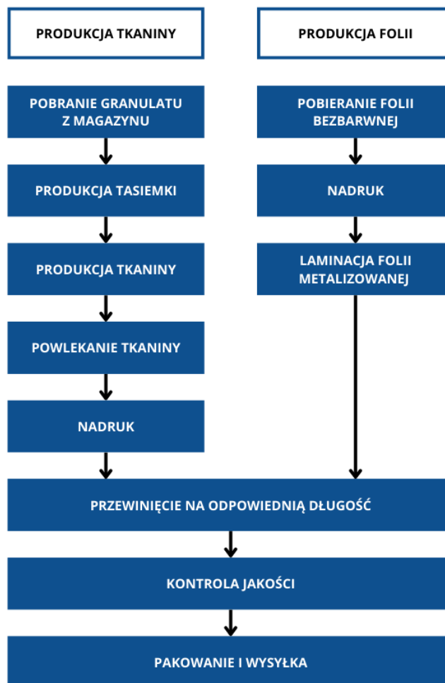
Rysunek 4.1: Uproszczony schemat produkcji folii i tkanin
