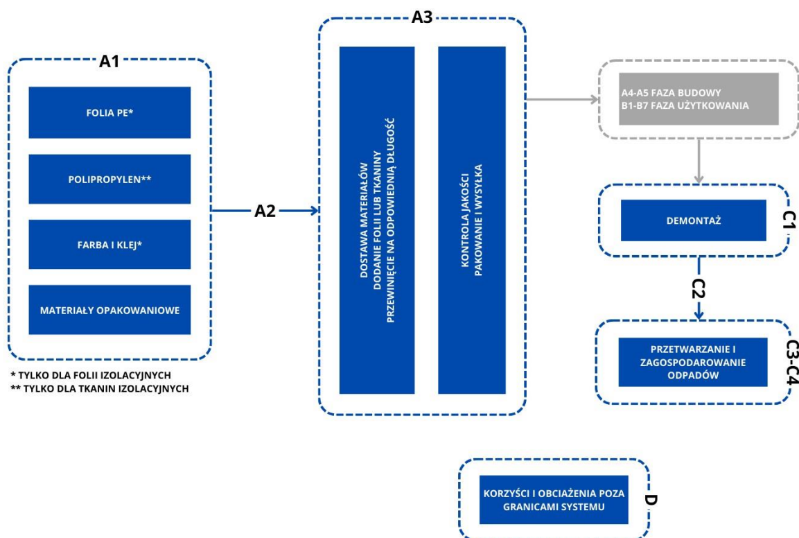
Rysunek 5.1: Granice systemu wykorzystane do charakterystyki środowiskowej
